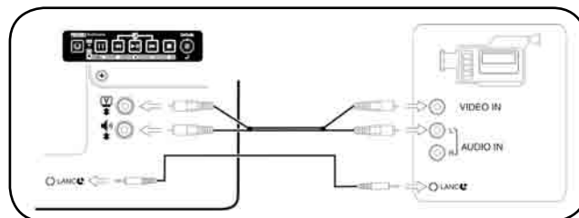
Управление внешним видеомэгнитофоном с приборной коробки цветного видеоприбора
